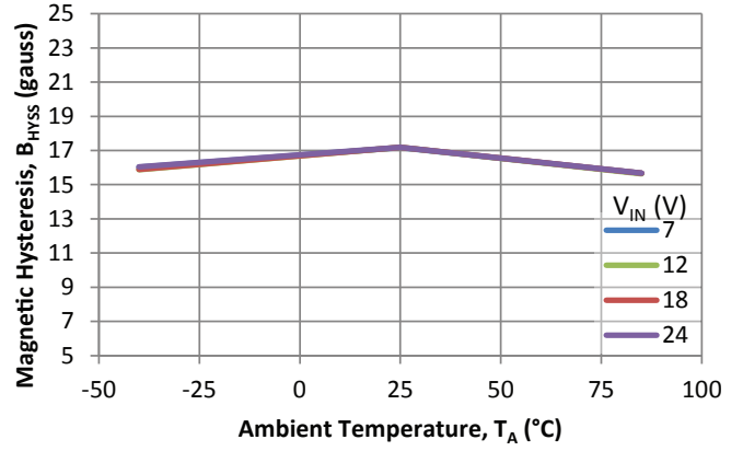
B_{HYSS} vs. T_A
